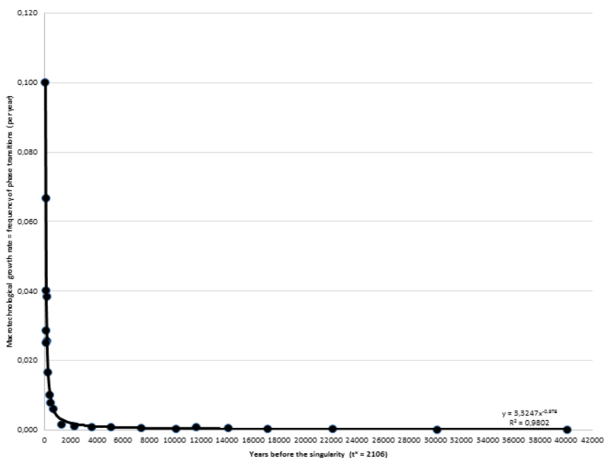
Рис. 7. Диаграмма рассеяния точек фазовых переходов (как эмпирически оцененных, так и прогнозируемых), описанных в Табл. 6, с подобранной степенной линией регрессии для даты сингулярности, определенной как 2106 г. методом наименьших квадратов (в натуральных цифрах)
