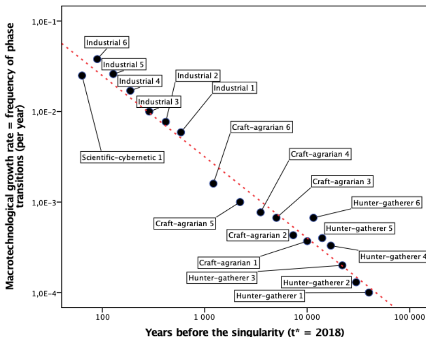
Рис. 6. Диаграмма рассеяния точек фазовых переходов, описанных в табл. 5, со встроенной линией степенной регрессии, где дата сингулярности определена как 2018 г. методом наименьших квадратов (двойная логарифмическая шкала)
