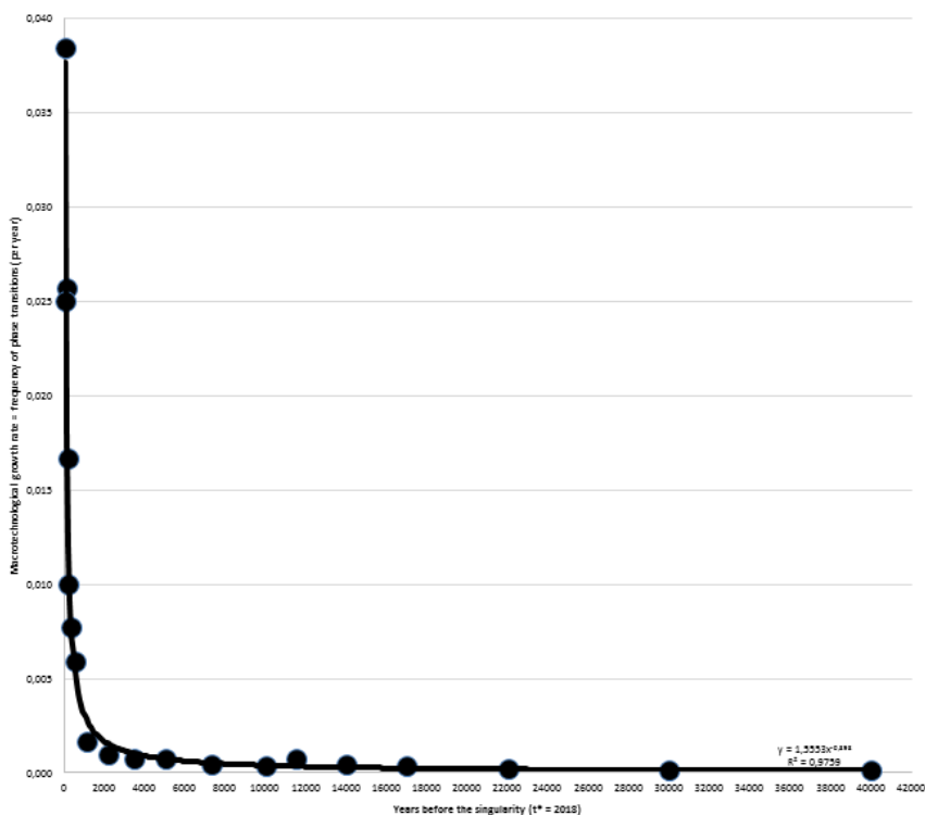
Рис. 5. Диаграмма рассеяния точек фазовых переходов, описанных в табл. 5, с подобранной степенной линией регрессии, где дата сингулярности определена как 2018 г. методом наименьших квадратов (натуральная шкала)
