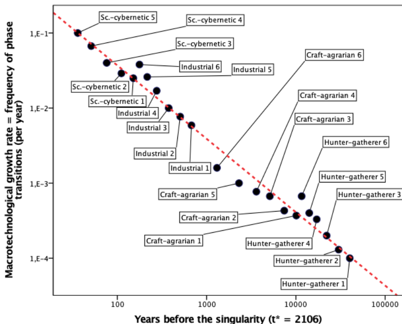
Рис. 8. Диаграмма рассеяния точек фазовых переходов (как эмпирически оцененных, так и прогнозируемых), описанных в табл. 6, с подобранной степенной линией регрессии для даты сингулярности, обозначенной как 2106 г. методом наименьших квадратов (двойная логарифмическая шкала)
