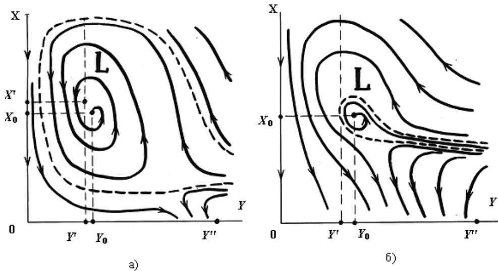
Рис. П21.9. Фазовый портрет автономных систем (29)–(30): а) низкие затраты на управление; б) высокие затраты на управление
