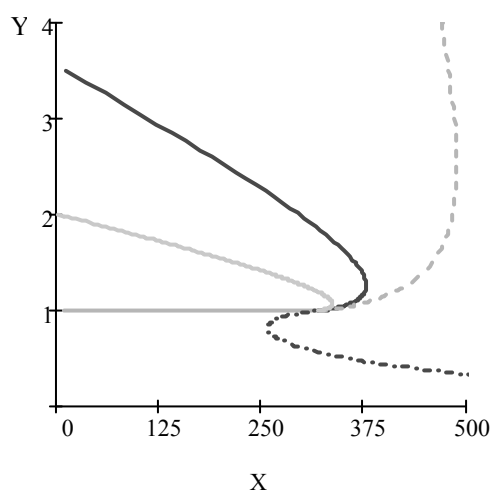
Рис. П21.1. Фазовые траектории системы (5) в координатах (Y, X)
