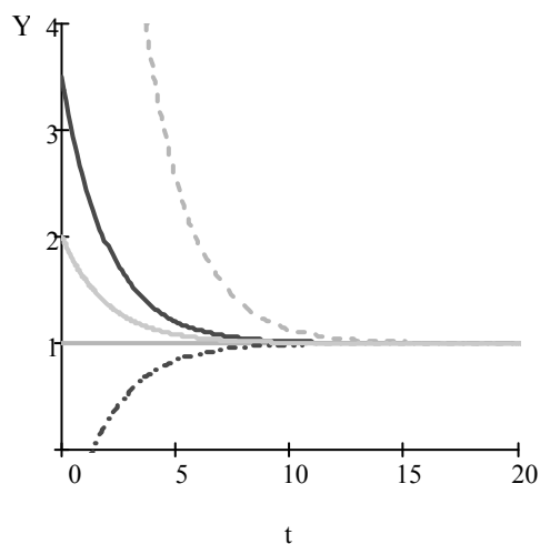
Рис. П21.2. Изменение величины средних накоплений земледельцев Y(t) (для различных начальных значений)
